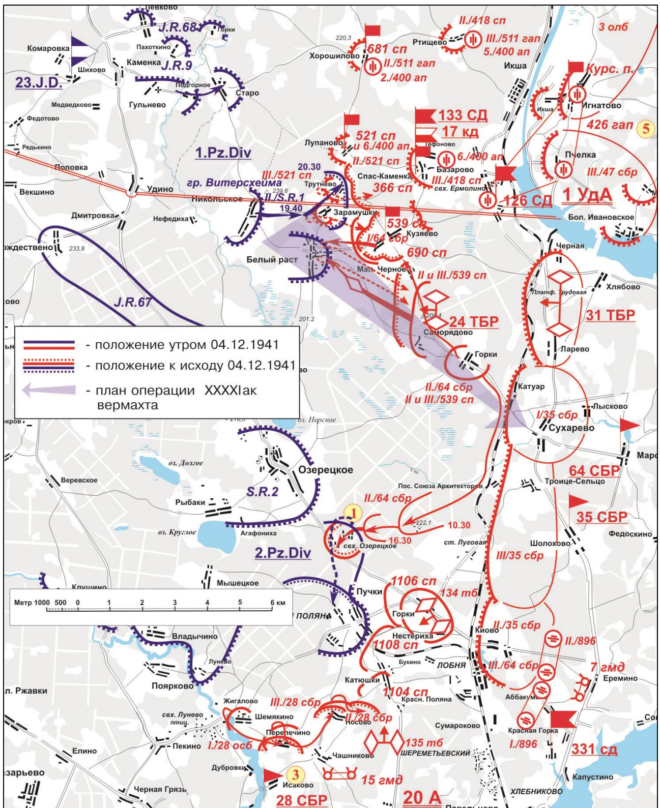
Положение на смежных флангах 1-й ударной и 20-й армий
